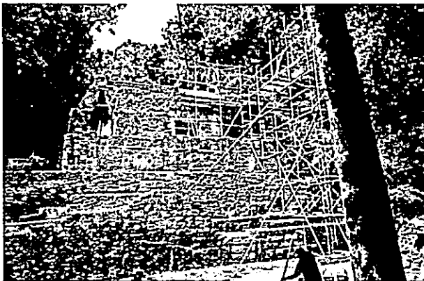
Figura No. 020. Edificio 375- Sistema de andamiaje construido para facilitar los trabajos
